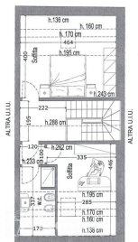
PIANTA PRIMO SOTTOTETTO (scala 1:100)
