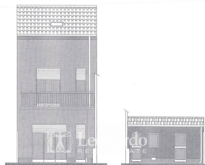
PROSPETTO RETRO (scala 1:50)
