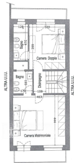
PIANTA PRIMO PIANO (scala 1:100)
