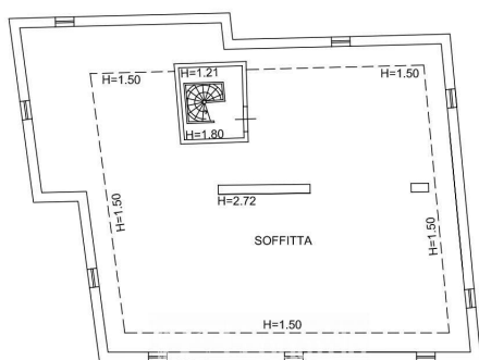
PIANO SECONDO
