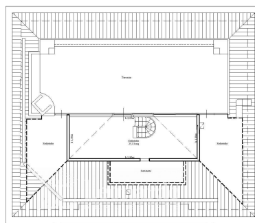
Pianta Piano Sottotetto
